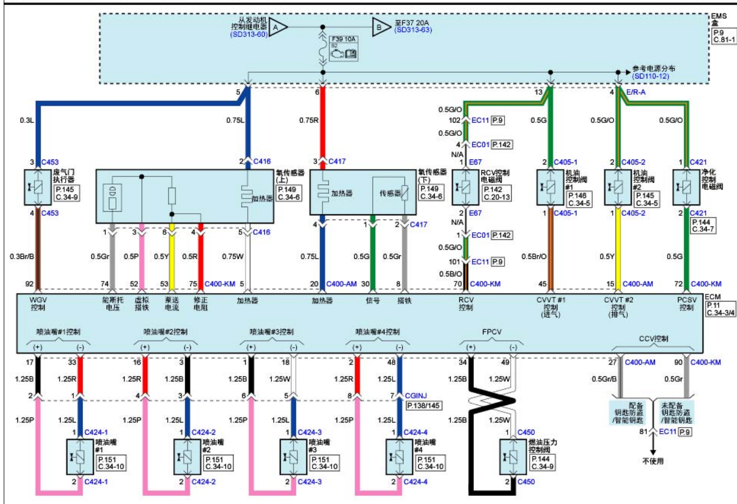
发动机控制系统(G4FJ: GAMMA 1.6L T-GDI M/T)(4)
